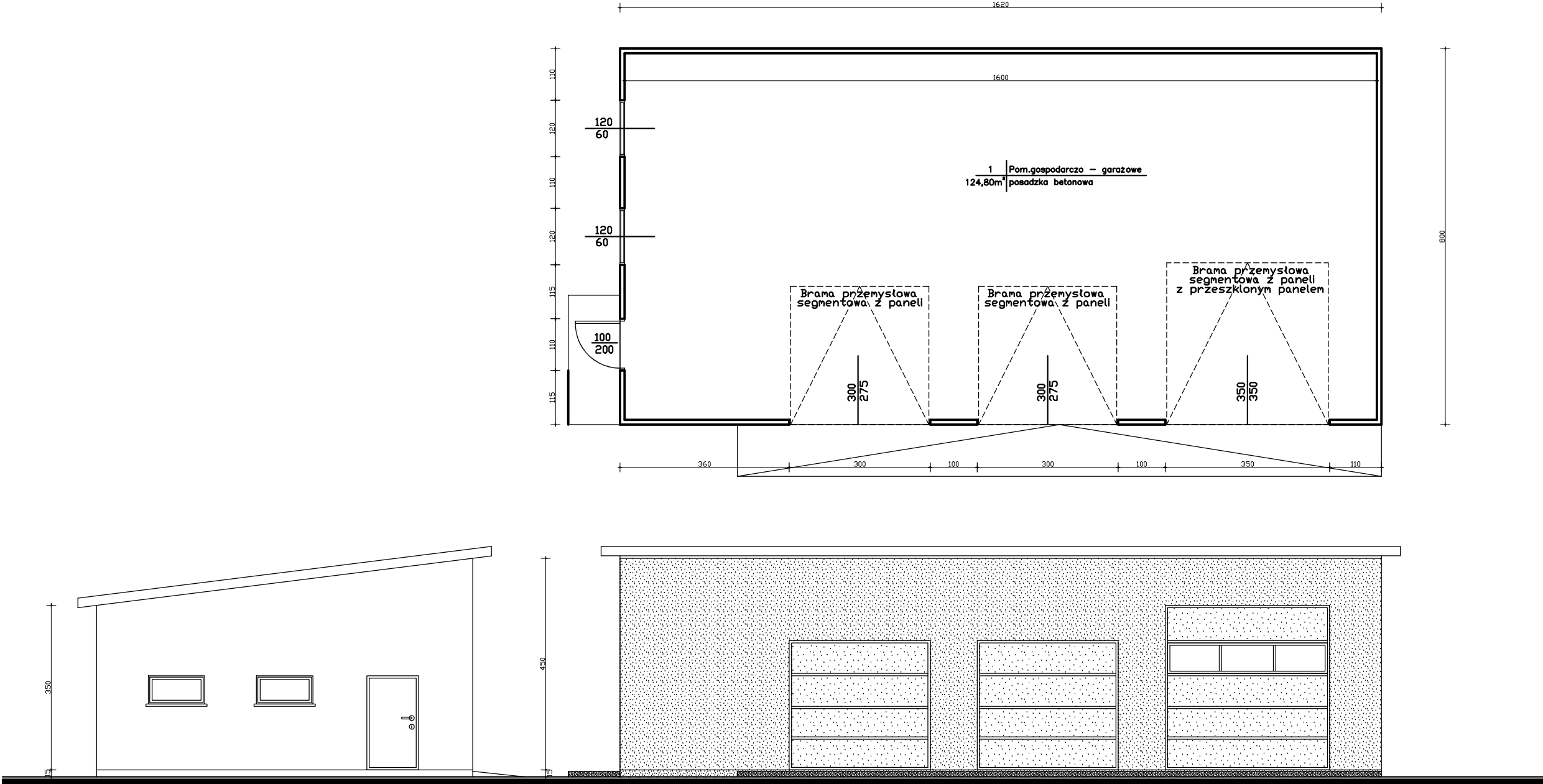
SCHEMAT POGLĄDOWY BUDYNKU GOSPODARCZO – GARAŻOWEGO
